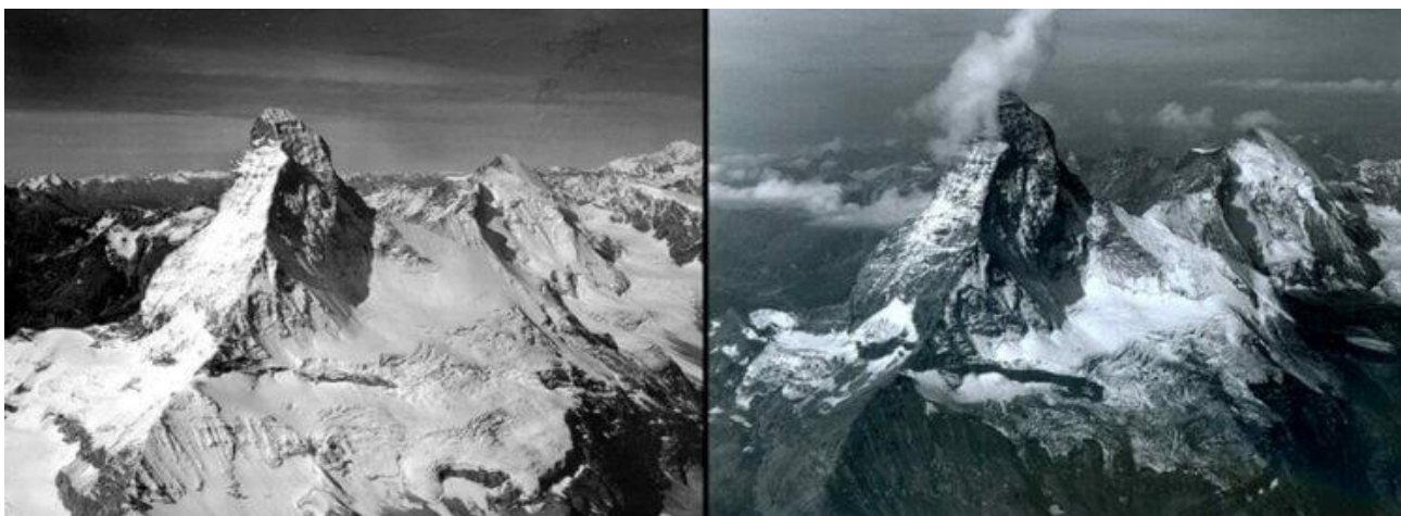
Рисунок 7 Пик Маттерхорн тогда и сейчас [53]
