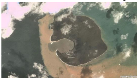
Рисунок 4 Вулканический остров Анак-Кракатау 30.12.2018 г. [50]
