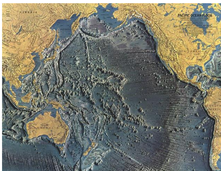
Рисунок 19 Космический снимок рельефа дна Тихого океана [40]
