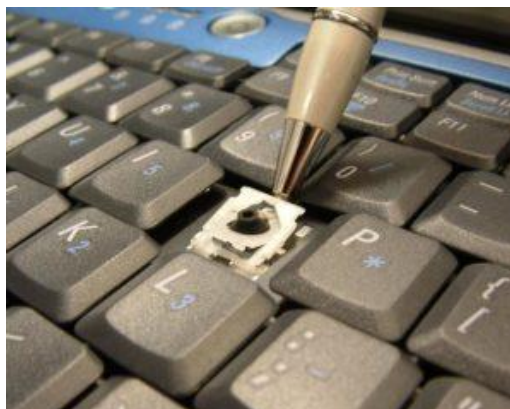
Рисунок 13 Ножничный механизм клавиатуры
