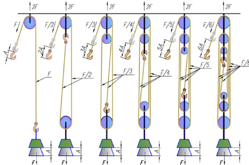
Рисунок 10 Полиспасты
